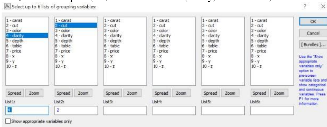
Рис. 24. Выбор переменных
